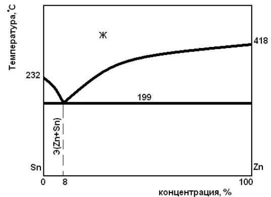
Рисунок А.8 – Диаграмма Sn-Zn
